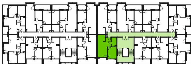
RZUT KONDYGNACJI 3
